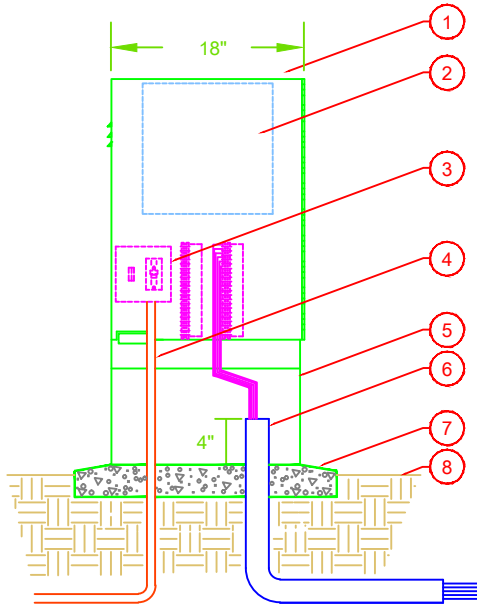
STRONGBOX DOUBLE DOOR ENCLOSURE
